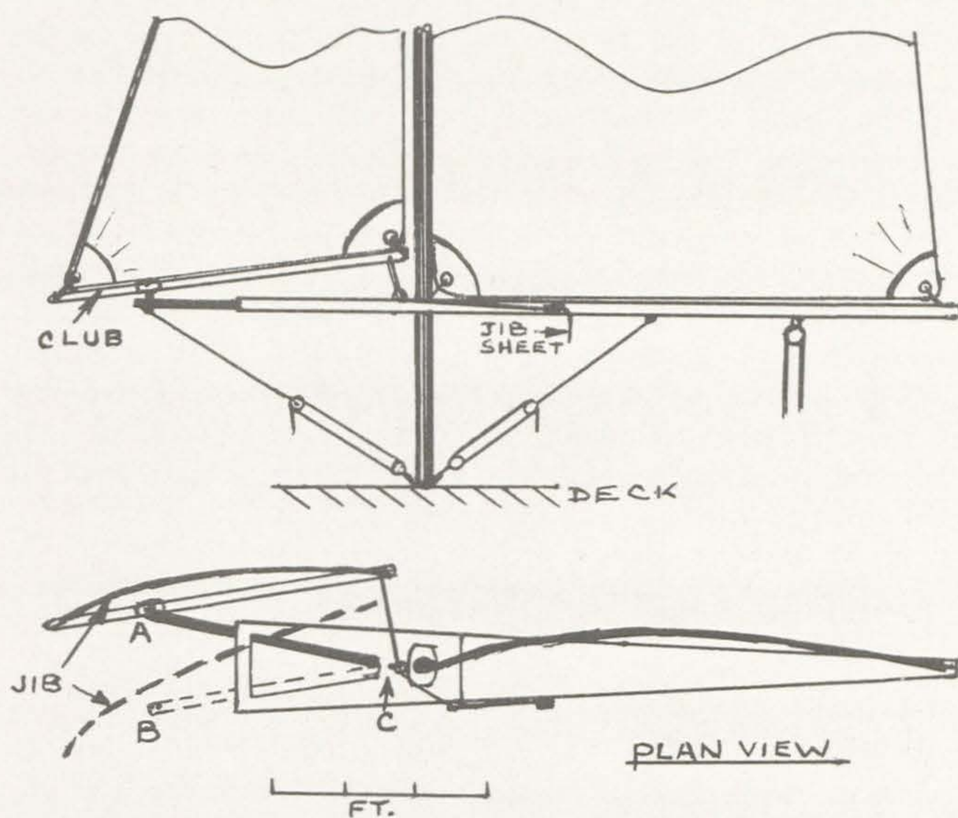
"BOOMSPRIT" RIG
