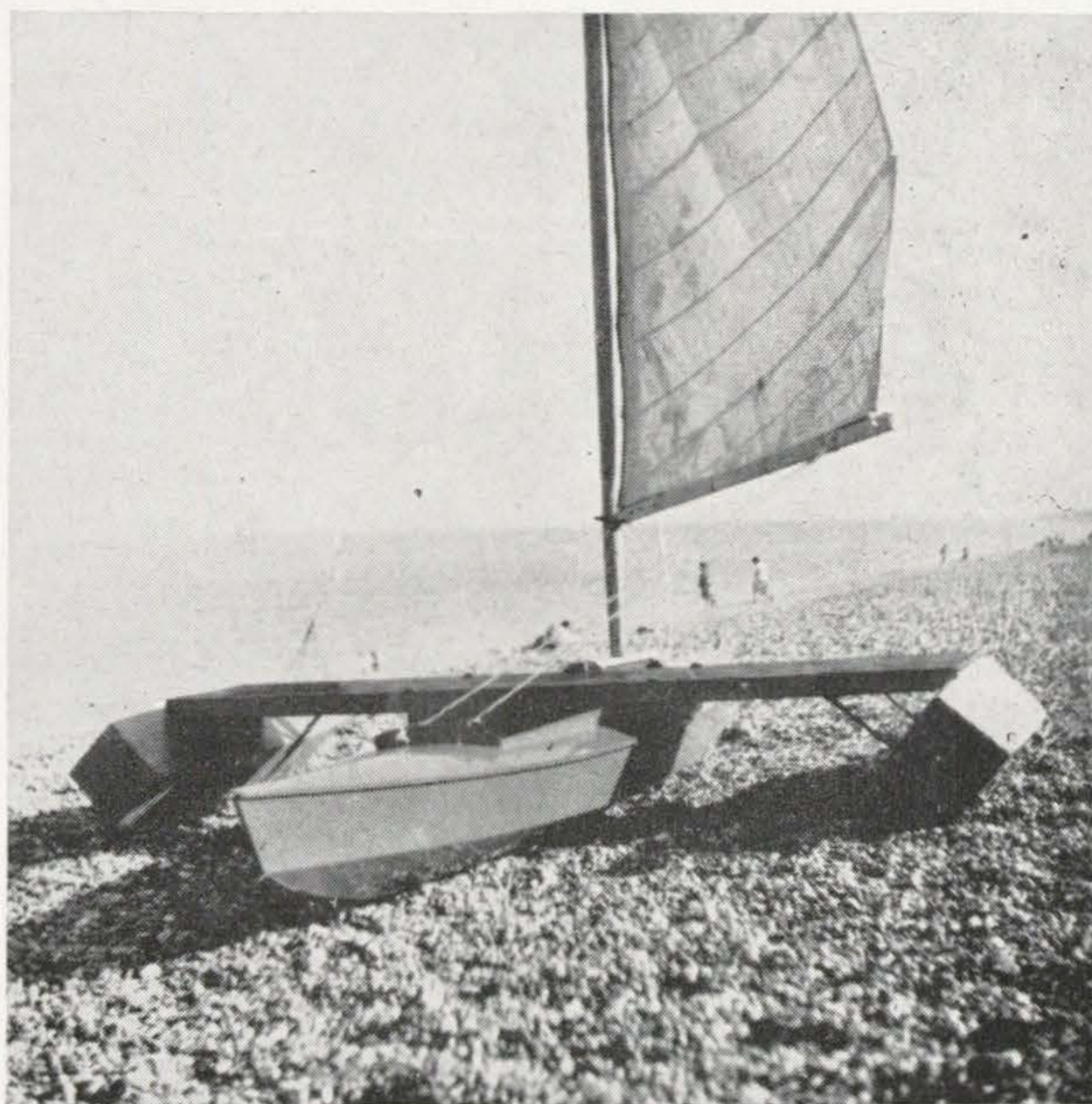
A miniature trimaran—J. Sidgwick
